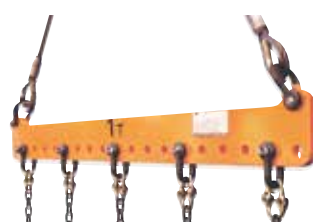
※LSB-900の吊金具
